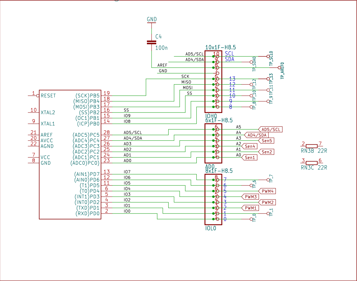
File: arduino_proiect.kicad_sch
