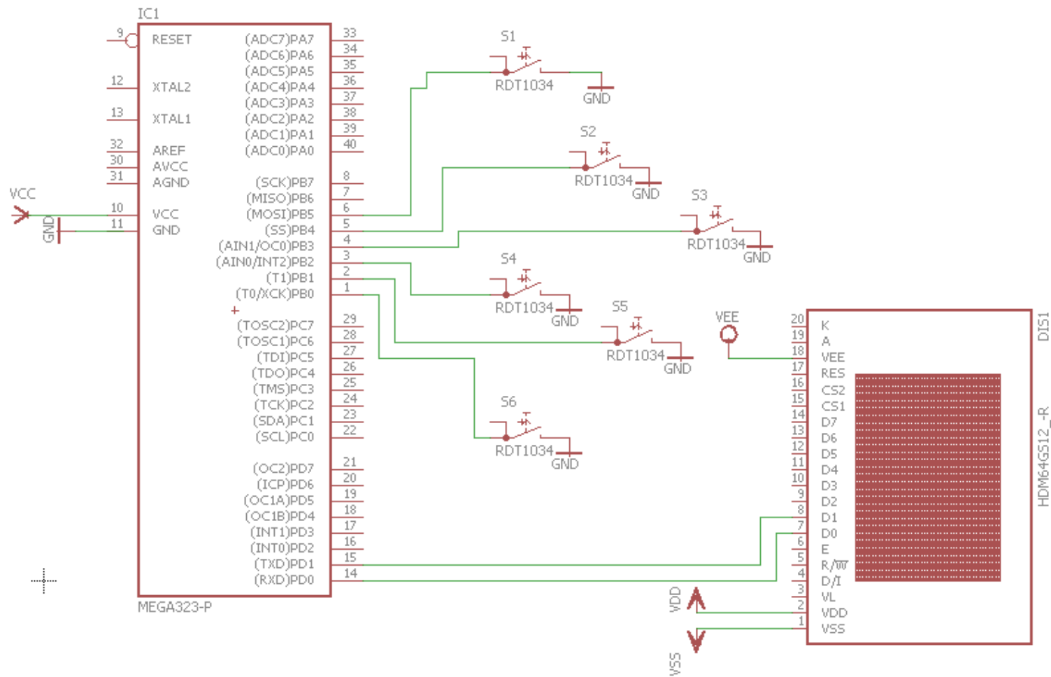
Schema electrica a proiectului Minesweeper:
