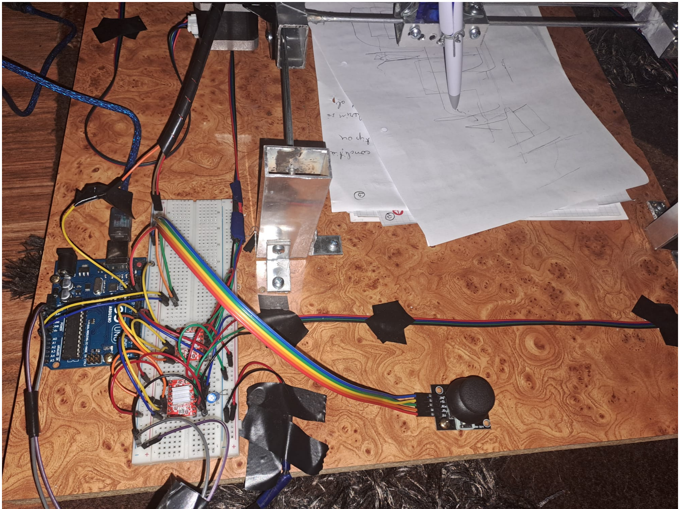
Aparatul intreg
