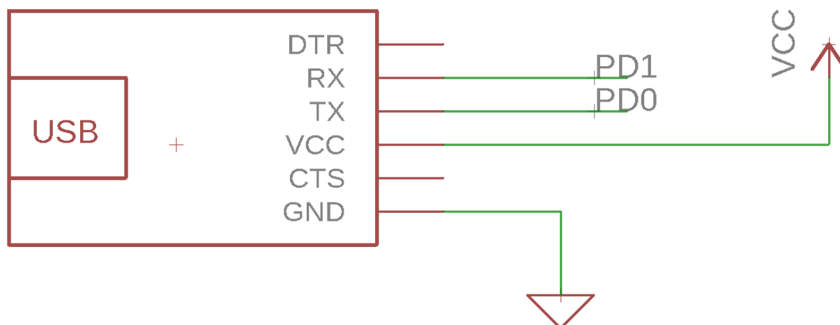
Schema FTDI
